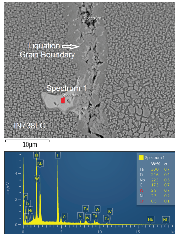
شکل ۱۷. آنالیز شیمیایی کاربید مرزانه MC ذوبی شده که به روش EDS شناسایی شده است
