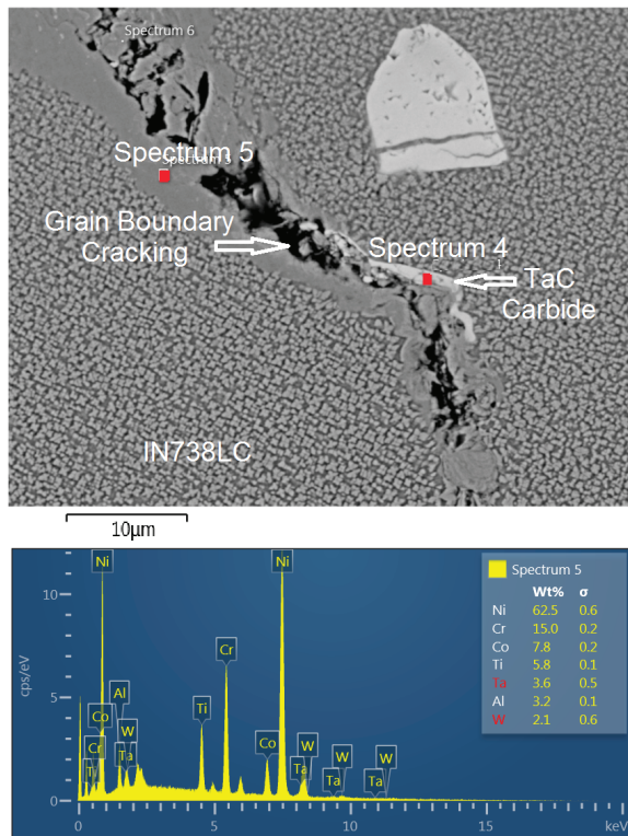
شکل ۱۸. آنالیز شیمیایی مرزانه دانه ذوبی شده سوپرآلیاژ IN738LC که به روش EDS اندازه‌گیری شده است
