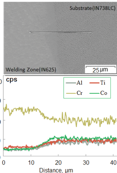
شکل ۱۲. تغییرات ترکیب شیمیایی عناصر W, Ti, Al, Cr و در ناحیه فصل مشترک فلز پایه با ناحیه لایه نشانی شده با لیزر
